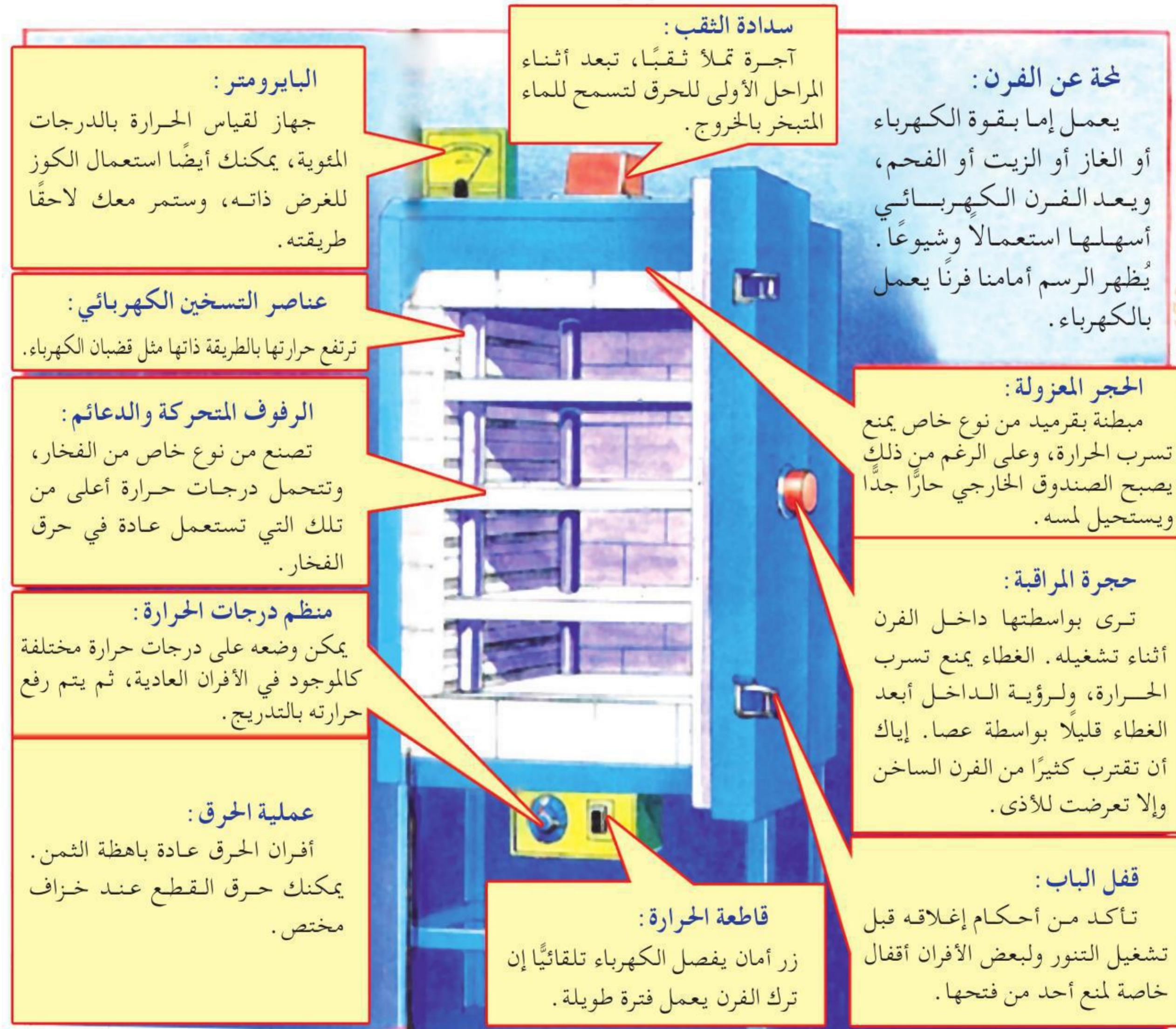
الشكل (٥٨): الأفران الحديثة أو الكهربائية والأجزاء التي تتكوّن منها.
